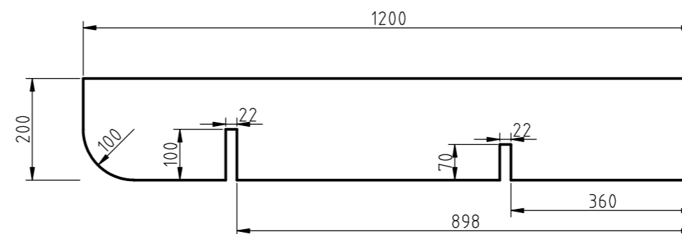
Teil 8, 9, 10, 11, Leimholz 18 mm
